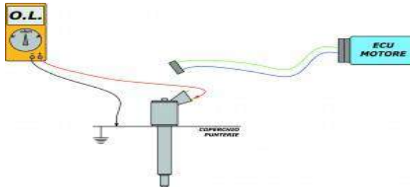
Izolimi i pinit 2 në anën e injektorit
