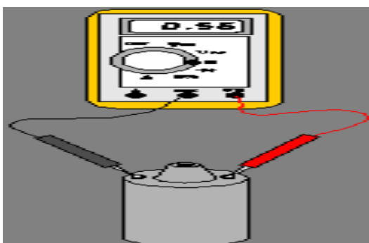
Matja e rezistencës PRIMARE
